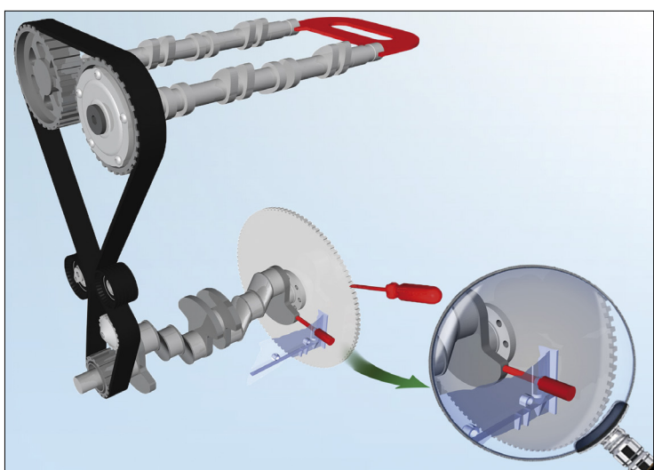
Slika 1: Pregled razvoda paljenja motora sa namještenom blokadom bregastih vratila, zatikom za osiguranje položaja koljenastog vratila i alatom za blokadu zamašnjaka (svi alati obojani su crveno).
