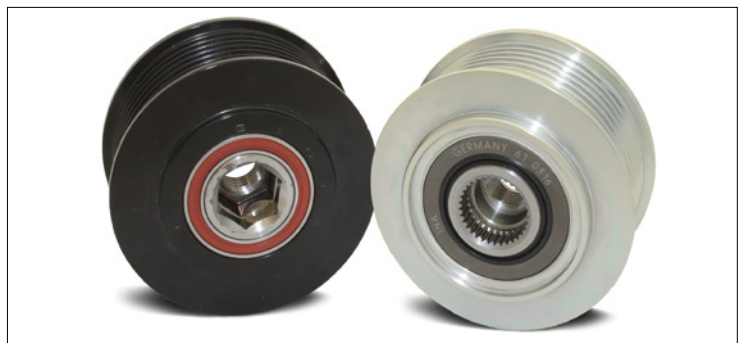
Photo 1: Poulie à roue libre d'alternateur réf. 535 0214 10
