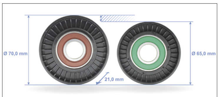
Fig. 2: Geleiderol 532 0404 30 voor voertuigen met benzinemotor (links) en geleiderol 532 0406 30 voor voertuigen met dieselmotor (rechts)
