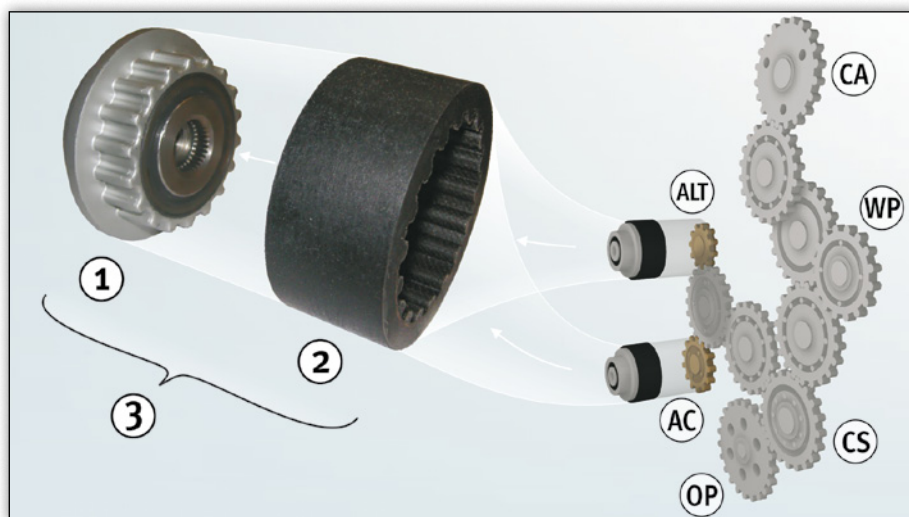
Fig. 1: Dynamovrijlooprol met flexibele koppelingsmof en tandwieloverbrenging met rechte vertanding
