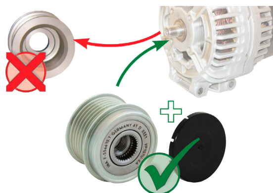
Bild 1: Utbyte av fast remskiva mot generatorfrinav
