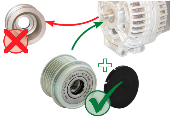
Kuva 1: Kiinteän hihnapyörän vaihto laturin vapaapyörään
