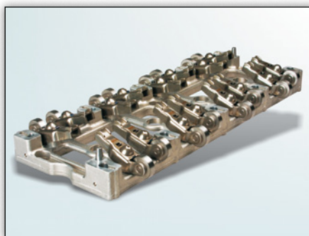
Figura 1: Telaio a bilanciere 423 0061 10
