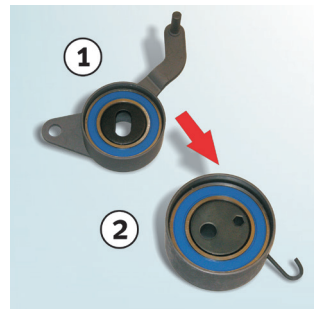
Зображення 1: Натяжний ролик 531 0166 20 (1) замінений на ролик 531 0819 10 (2)
