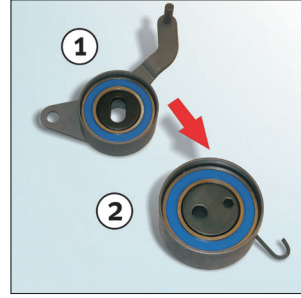
Resim 1: Eski gergi rulmanı 531 0166 20 (1) ve yeni gergi rulmanı 531 0819 10 (2)
