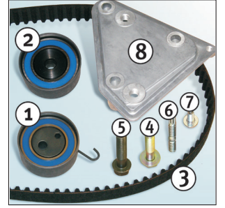
Resim 2: Paket içeriği: 530 0492 10
