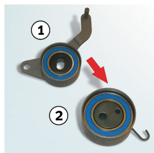
Figur 1: Erstattet spennrulle 531 0166 20 (1) og dens etterfølger 531 0819 10 (2)
