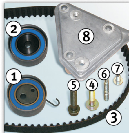
Figura 2: Contenuto della confezione 530 0492 10
