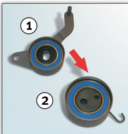
Figura 1: Rullo tenditore sostituito 531 0166 20 (1) e successivo 531 0819 10 (2)
