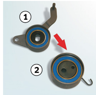
Kuva 1: 1. Korvattu hihnankiristin 531 0166 20 2. Uusi hihnankiristin 531 0819 10
