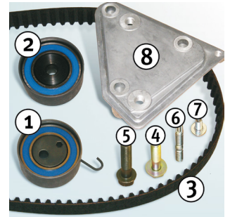
Kuva 2: INA KIT 530 0492 10
