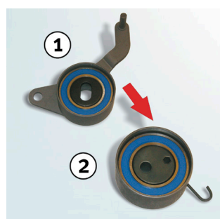
Billede 1: Erstattet strammerulle 531 0166 20 (1) og dens efterfølger 531 0819 10 (2)
