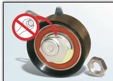
Slika 2: Šesterorobi okov na zadnji strani napenjalne jermenice nima nobene funkcije
