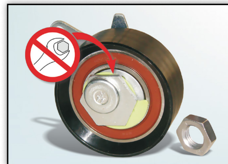
Slika 2: Šesterorobi okov na zadnji strani napenjalne jermenice nima nobene funkcije
