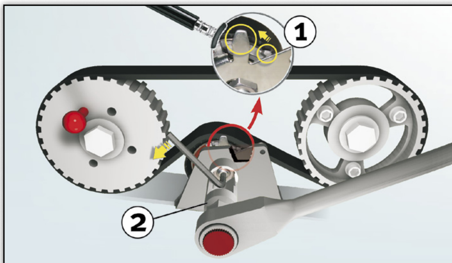
Fig. 1: Aandrijvings- en positieoverzicht voor spanrol en speciaal gereedschap
