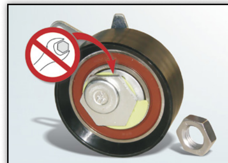
Fig. 2: De zeskant op de spanrol heeft geen functie
