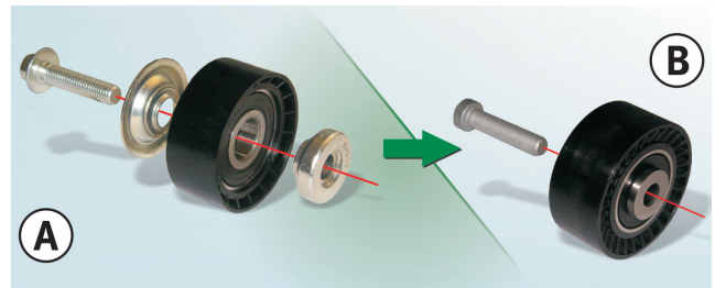
Зображення 1: Обвідний ролик 532 0433 10, попередня версія (A) і нова версія (B)
