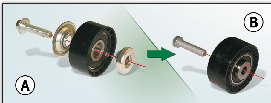
Preusmerjevalni valj 532 0433 10, dosedanja izvedba (A) in nova izvedba (B)
