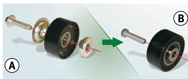
Rolă deflectoare 532 0433 10, design precedent (A) și design nou (B).
