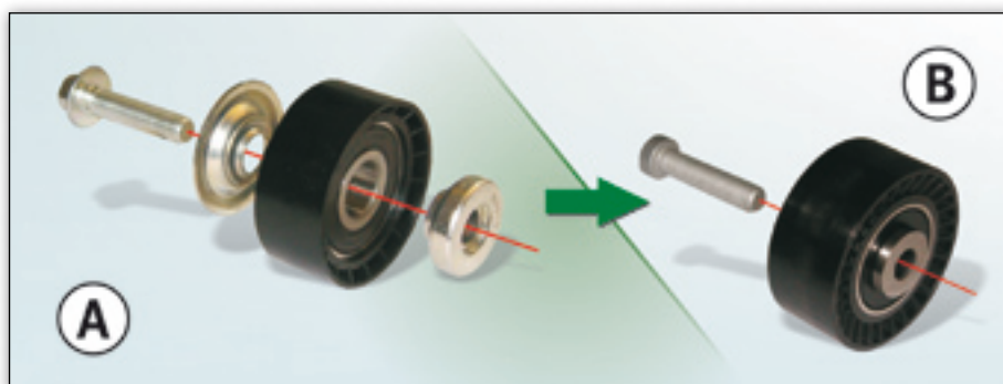
Geleiderol 532 0433 10, bestaande uitvoering (A) en nieuwe uitvoering (B)
