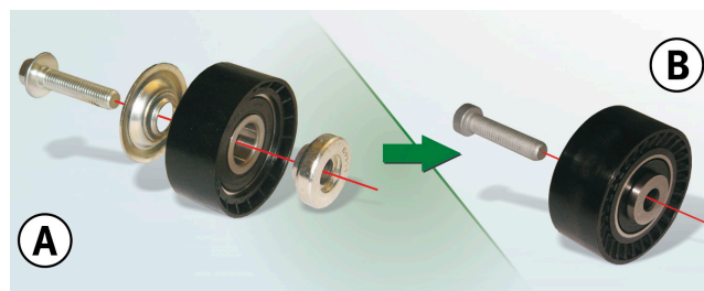
532 0433 10 számú vezetőgörgő, eddigi kivitel (A) és az új kivitel (B)
