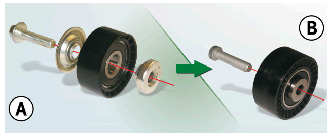
Τροχαλία 532 0433 10, παλιός (Α) και νέος σχεδιασμός (Β)
