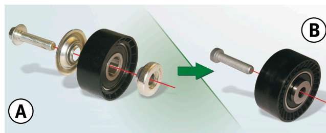
Снимка 1: Отклоняваща ролка 532 0433 10, предишен модел (A) и нов модел (B)
