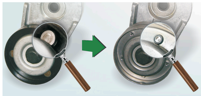
1. ábra: A futógörgők eddigi kivitelének (bal) és az új kivitelek (jobb) részletes nézete
