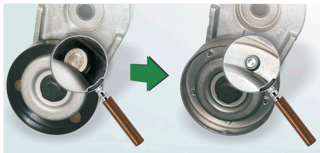
Εικόνα 1: Λεπτομερής προβολή των τροχαλιών στην έκδοση που υπήρχε μέχρι τώρα (αριστερά) και στη νέα έκδοση (δεξιά)
