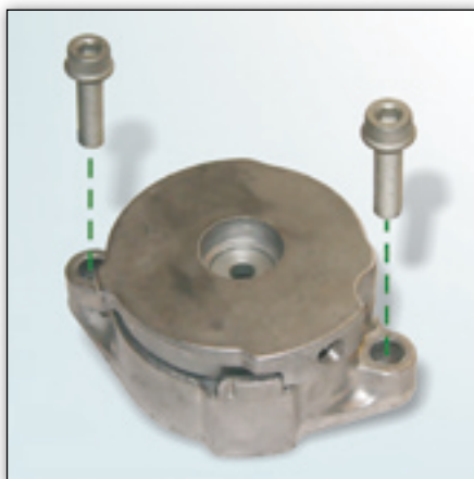
Fig. 1: INA-uitvoering met twee schroeven M8x35
