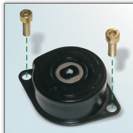
Image 2 : Version avec deux vis M8 x 22
