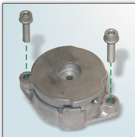
Image 1 : Version INA avec deux vis M8 x 35
