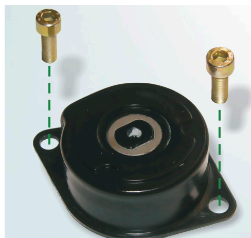
Billede 2: Specifikation med to skruer M8x22
