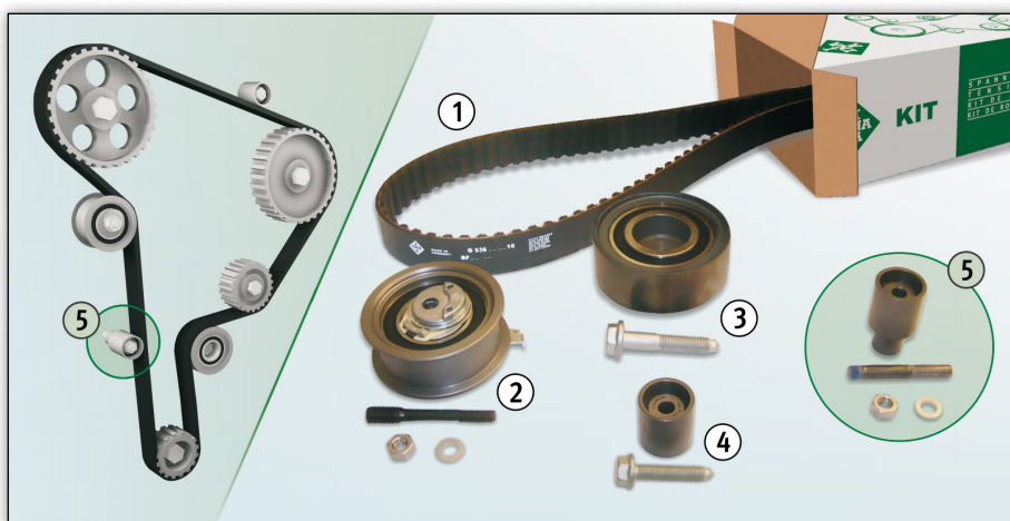
Slika 1: Dijagram vođenja remena kod 1.9 TDI/SDI i sadržaj kitova Kat. Br. 530 0361 10/530 0082 10
