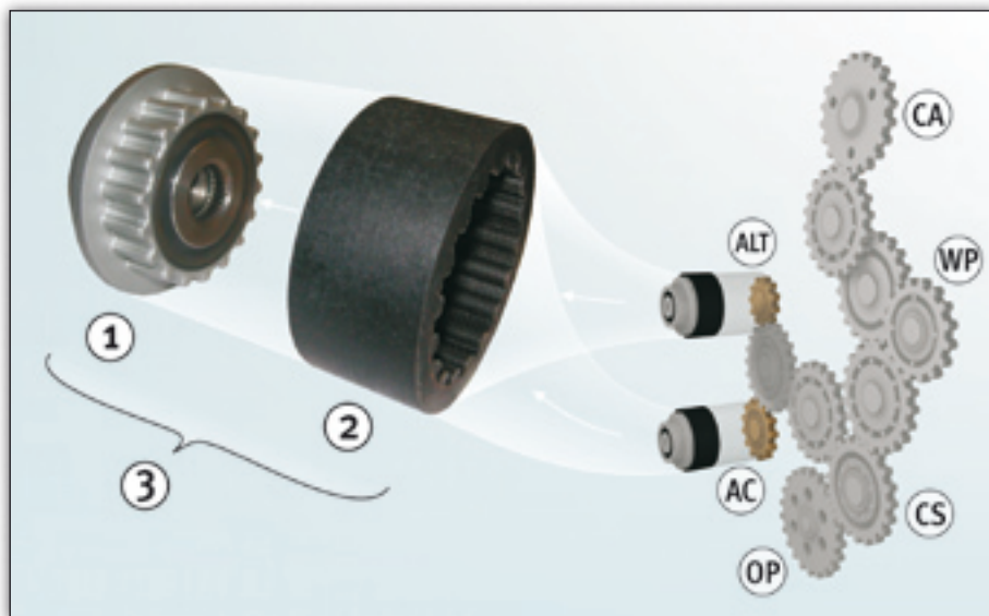
Figuur 1: Generatorvrijlooprol met flexibele koppelingsmof en tandwieloverbrenging met rechte vertanding
