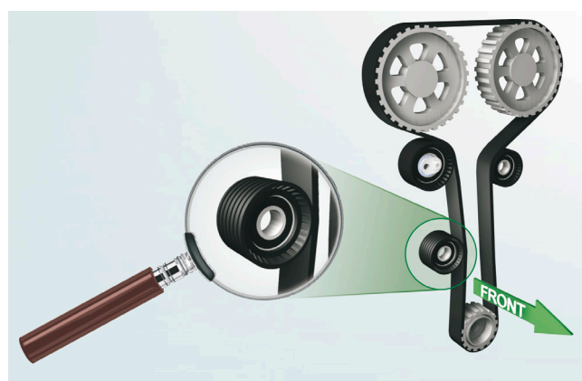
Billede 1: Remmens forløb og rullepositioner i F4R-motoren
