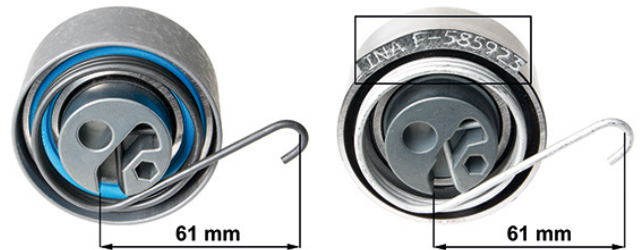
Зображення 1: 531 0535 20 — стара версія (зліва), нова версія (справа)
