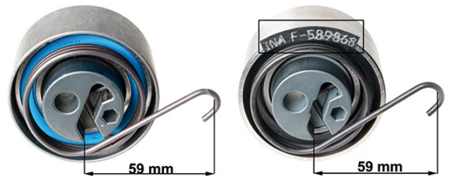
Зображення 2: 531 0819 10 — стара версія (зліва), нова версія (справа)
