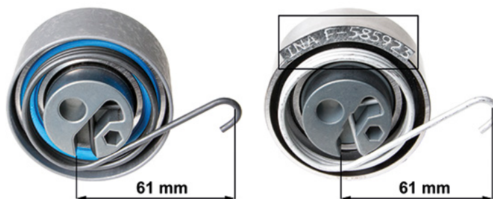
Slika 1: 531 0535 20 – stara izvedba (lijevo), nova izvedba (desno)
