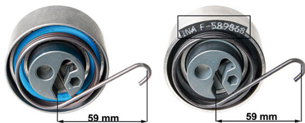
Εικόνα 2: 531 0819 10 – παλιός σχεδιασμός (αριστερά), νέος σχεδιασμός (δεξιά)
