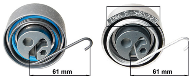
Εικόνα 1: 531 0535 20 – παλιός σχεδιασμός (αριστερά), νέος σχεδιασμός (δεξιά)
