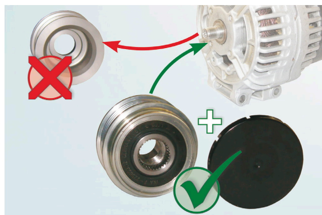
Obrázek 2: Výměna alternátorové volnoběžky
