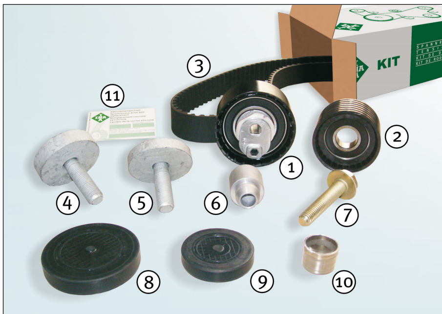
Slika 1 – kompletan sadržaj seta s razvodnim remenom - INA KIT 530 0363 10
