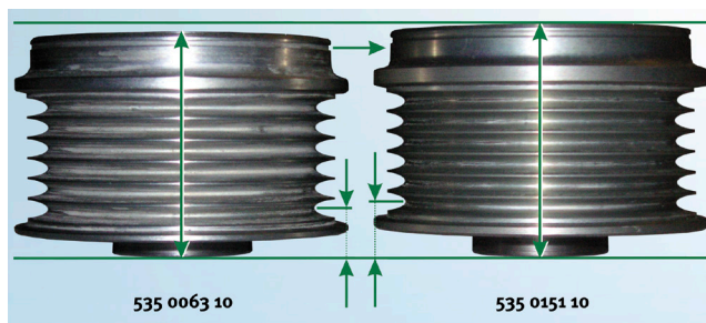
Зображення 3: Відмінність між шківами генератора з обгінною муфтою INA 535 0063 10 (VALEO) і 535 0151 10 (DENSO)
