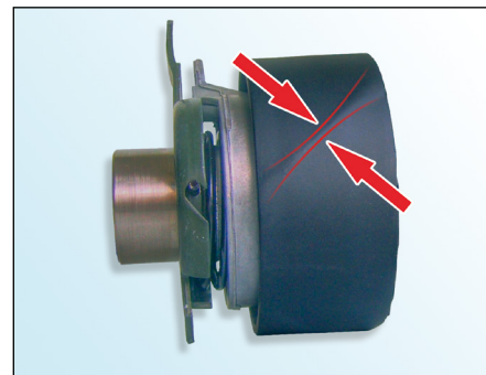
Slika 2: 531 0564 30 (pogled od strani)
