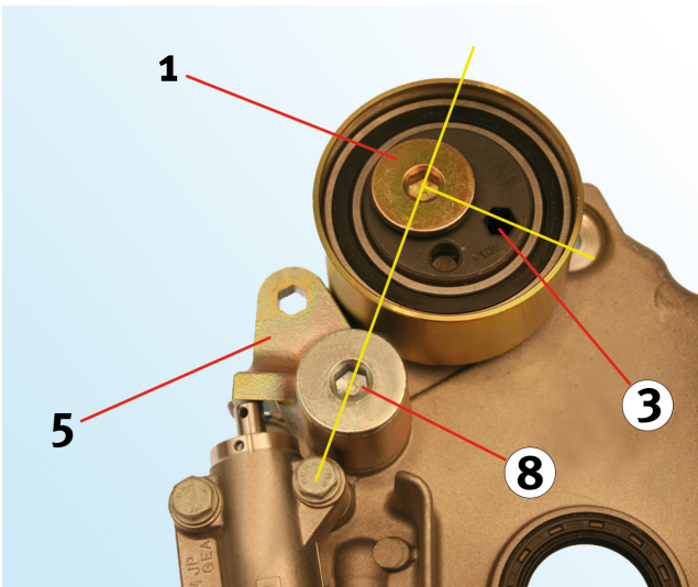
Bild 4: Korrekt monteringsposition (sedd framifrån).
