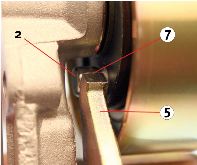
Bild 3: Korrekt monteringsposition (sedd bakifrån).
