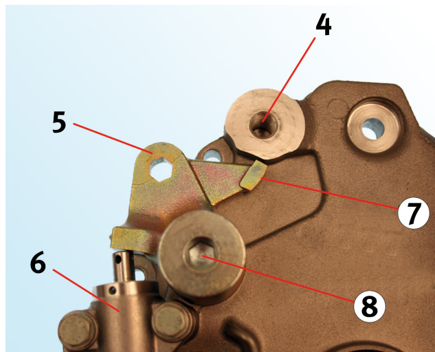
Bild 2: Lagarsköld till vevaxel
