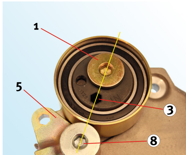
Bild 6: Felaktig monteringsposition (sedd framifrån).
