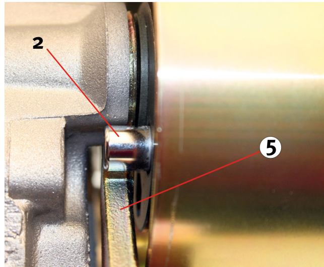
Bild 5: Felaktig monteringsposition (sedd bakifrån).
