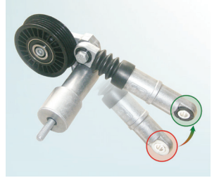
Resim 2: 534 0014 10 - Hidrolik sönümleyicideki siyah ve beyaz plastik burçları gösteren versiyon
