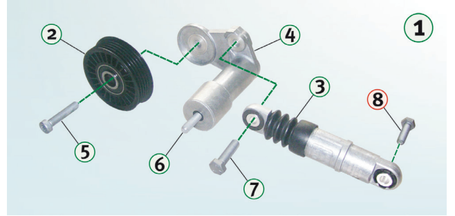
Resim 1: Tüm bileşenleriyle beraber 534 0014 10'un ayrıntılı çizimi
