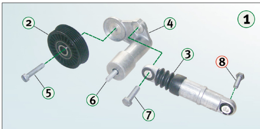
Fig. 1: Representación detallada de 534 0014 10 con todos los componentes
