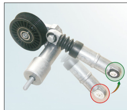
Fig. 2: 534 0014 10 - Versión con anillos sintéticos blancos y negros en el amortiguador hidr.
