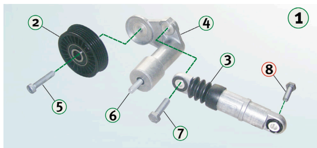
Фигура 1: Подробна илюстрация на 534 0014 10, включваща всичките му компоненти
