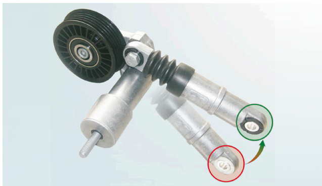
Фигура 2: Версия 534 0014 10, като са показани както черните, така и белите пластмасови втулки на хидравличния демпфер
