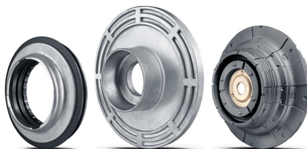
Bild 1: Federbeinstützlager (Einzellager, geschmiedeter Teller und TopMount)
