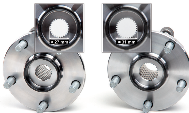
Fig. 2: De diameter van de aandrijfasopname is verschillend
