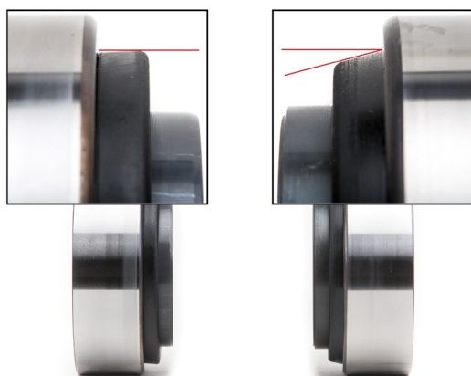
1 pav. Pakeista apsaugos nuo dulkių konstrukcija
