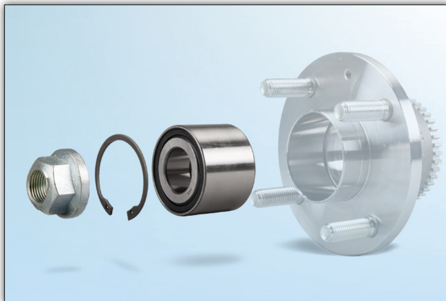
Fig. 1: De FAG-wiellagerset 713 6448 00 als reparatieoplossing: de wielnaaf hoeft hierbij niet te worden vervangen.
