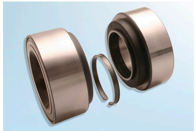
Зображення 1: Ремонтний вузол ступиці (RIU)
