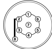
Johtojen liittäminen 7-napaiseen pistorasiaan
