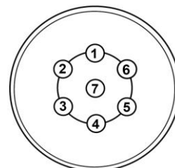
Tilkobling av ledninger i den 7-polete kontakten
