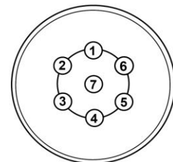
Johtojen liittyminen 7-nappaiseen pistorasiaan
