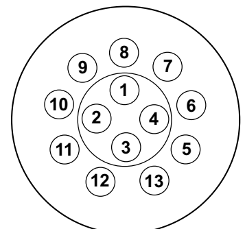
Kontaktbelegung der Steckdose
