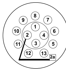
Connecteur des câbles le jack à 13 pôles
